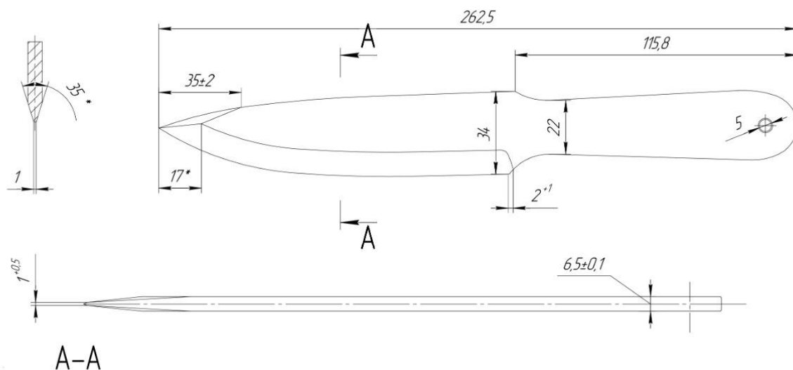
Рисунок № 8. Ножи для метания «СМН».
