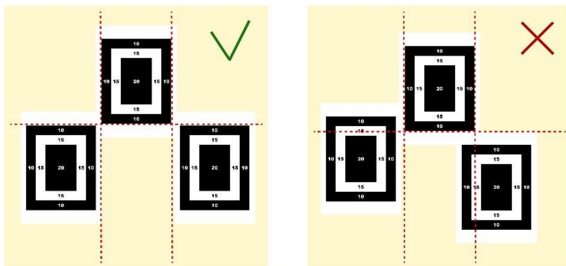
Рисунок №6. Расположение мишеней на стенде.
