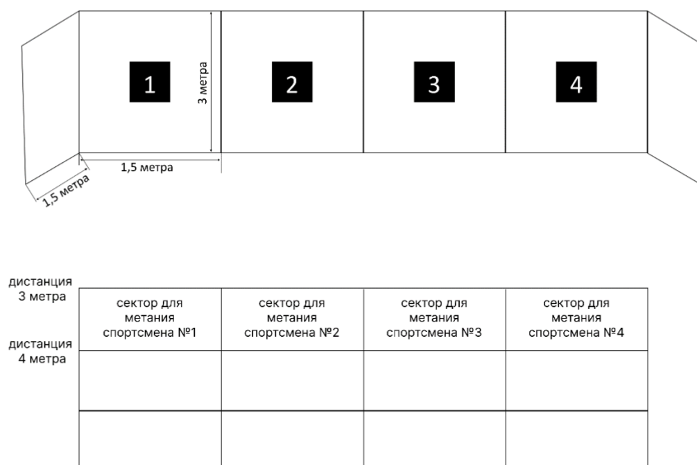
Рисунок № 2. Защитная стена для стендов и сектора для метания.
